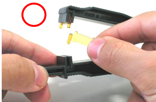
(良い例) 斜めにカッティングされている方が上
