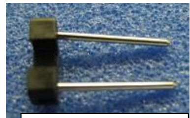
把持部材付き勸合ピン
